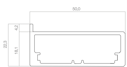
ALUPROFIL TYP SAS088 OBERFLÄCHE: AL1 - ALU NATUR MATT
