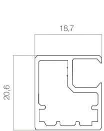
ALUPROFIL TYP SAS001 OBERFLÄCHE: AL1 - ALU NATUR MATT EE - EDELSTAHL
