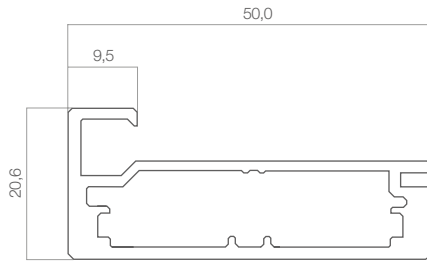
ALUPROFIL TYP SAS077 OBERFLÄCHE: AL1 - ALU NATUR MATT EE - EDELSTAHL
