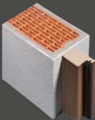
BLENDRAHMEN BM 43/65 in der Laibung montiert (beliebige Position)
