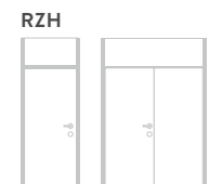
Raumhohe Zarge ohne Querteil mit Kämpfer und Oberlichte bis Raumlichte von 2.600 mm (einflügelig, zweiflügelig)
