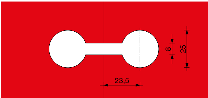
ANSICHT AUSFRÄSUNGEN FÜR KUPPLUNG
