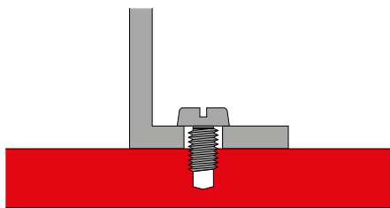
VERBINDUNG MIT GEWINDEBOHRUNG DIREKT IN DIE COMPACTPLATTE
