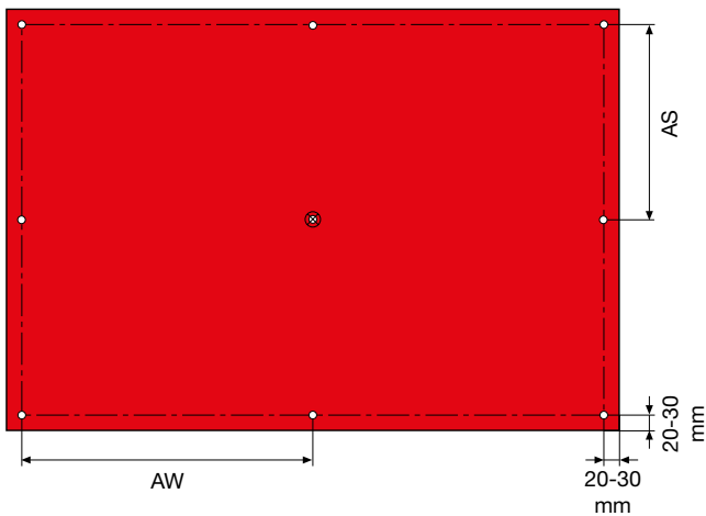
BEFESTIGUNGSABSTÄNDE ⊗ FIXPUNKT
