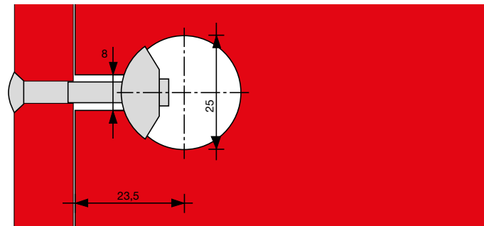
SEITENANSICHT KUPPLUNGSBOHRUNG
