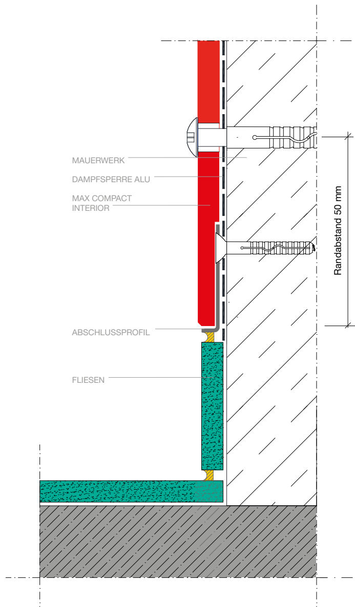
LOTSCHNITT RAMMSCHUTZ - BODENANSCHLUSS BÜNDIG MIT FLIESEN
