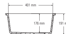
QUERSCHNITT SEITENANSICHT
