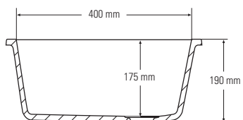
QUERSCHNITT SEITENANSICHT
