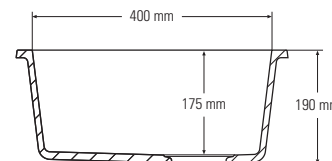
QUERSCHNITT SEITENANSICHT
